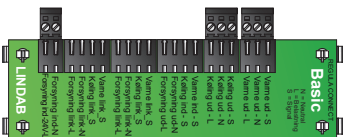
Billede 3. Weidmüller 1 x 2-pole-hun (670290) og 2 x 3-pole-hun (670291).
