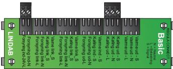
Billede 2. Weidmüller 1 x 2-pole-hun (670290) og 1 x 3-pole-hun (670291).
