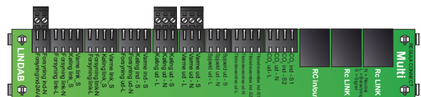
Billede 6. Weidmüller 1 x 2-pole-hun (670290) og 2 x 3-pole-hun (670291).
