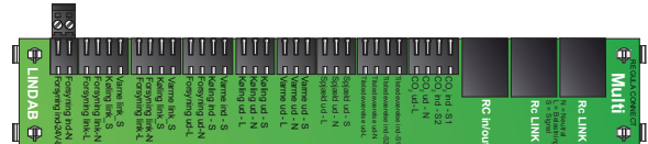
Billede 4. Weidmüller 2-pole-hun (670290).
