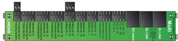
Billede 5. Weidmüller 1 x 2-pole-hun (670290) og 1 x 3-pole-hun (670291).
