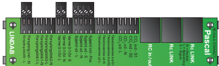
Billede 8. 2 x Weidmüller 2-polet hun (en til strømforsyning, altid inkluderet) og 1 x 3-polet hun. Se Billede 8.B "eksempel fra kabelskemakonfiguratoren".
