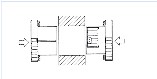
Figur 2, montasjeprinsipp
