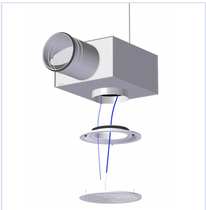
Figur 5, montasje
